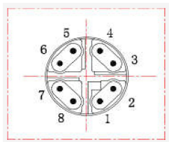
M12 X编码8芯公头孔位图
